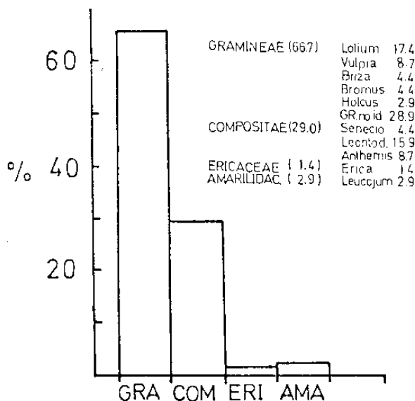
Fig. 1. Frecuencia relativa de aparición de las familias y géneros de plantas observadas por análisis microscópico de las pelotas fecales de los conejos de Martinazo. Junio, 1977. Reserva Biológica de Doñana. S.O. España.
